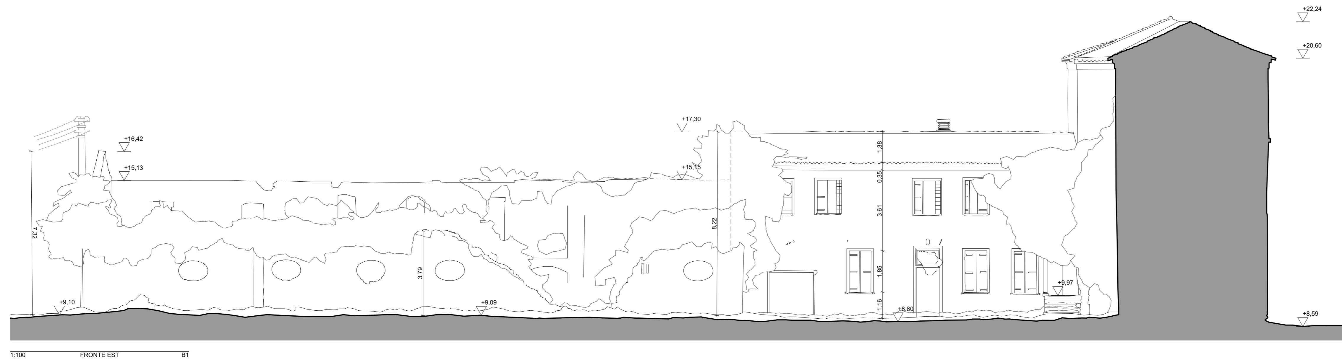
1:100 FRONTE EST B1
